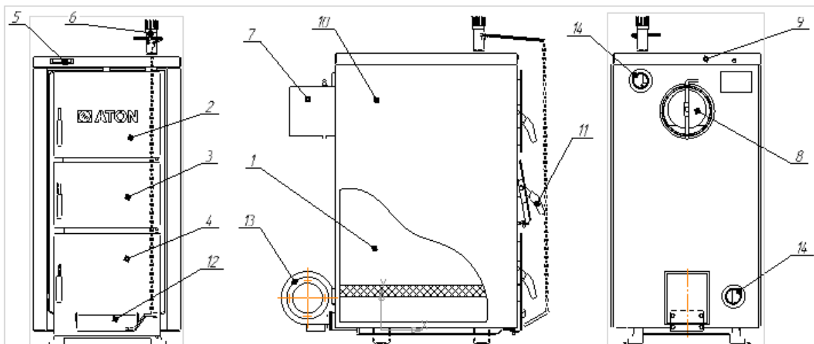
Малюнок 1. Котел опалювальний ATON TTK Multi
