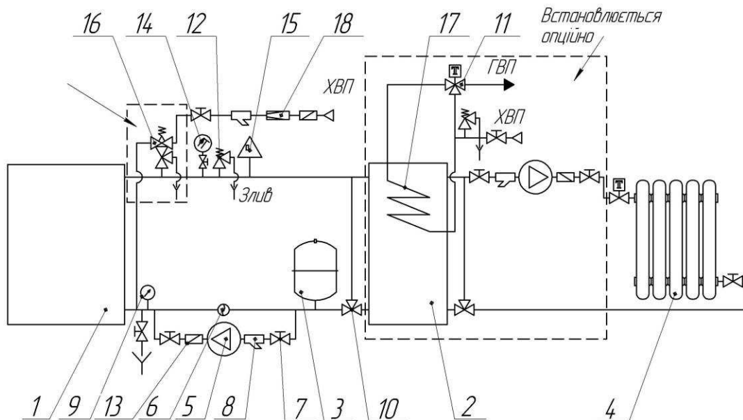
Малюнок 5. Схема підключення котла до закритої системи опалення з примусовою циркуляцією 1 - котел; 2 - буферна ємність (теплоакумулятор); 3 - мембранний бак; 4 – радіатор; 5 - циркуляційний насос; 6 - диференціальний клапан; 7 - кран шаровий; 8 - фільтр грубої очистки; 9 – термометр; 10 – термостатичний підмішувальний клапан; 11 - термостатичний 3-х ходовий клапан; 12 - клапан безпеки (2 bar); 13 - зворотній клапан; 14 - термоманометр з спускний краном; 15 – повітрявідвідник; 16 - клапан безпеки термостатичний Regulux DBV 1-02; 17 – змієвик; 18 - клапан редукційний.
